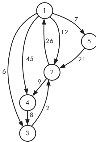
Рис. 5.1. Граф мышиного лабиринта
