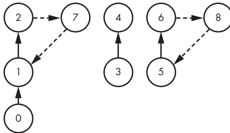
Рис. 8.9. Структура данных после еще одной операции SetEnemies
